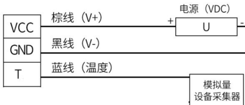
模拟量接线示意图
