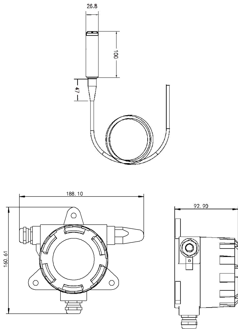
尺寸图 (单位: mm)
