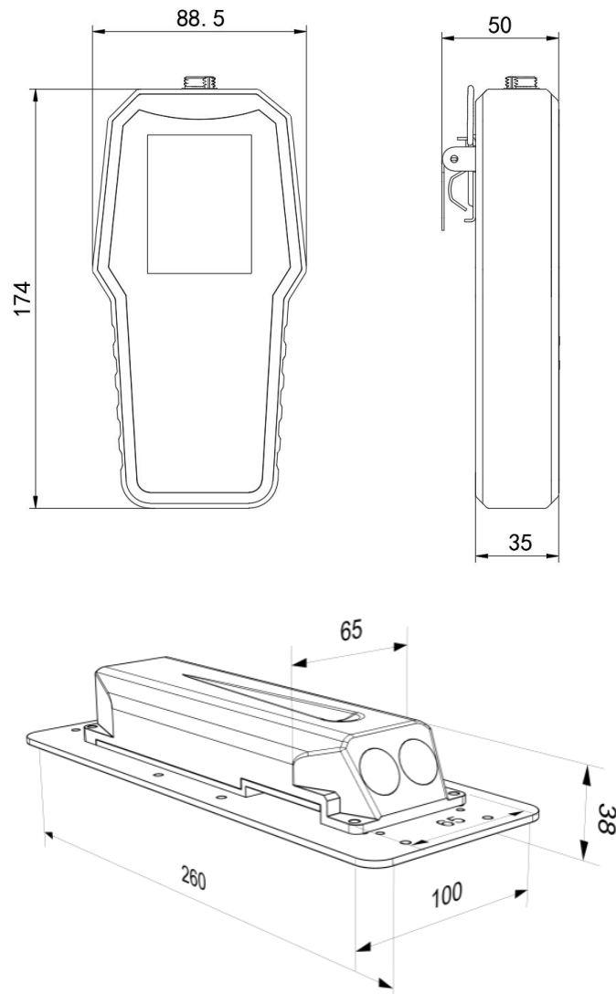
设备尺寸图（单位：mm）
