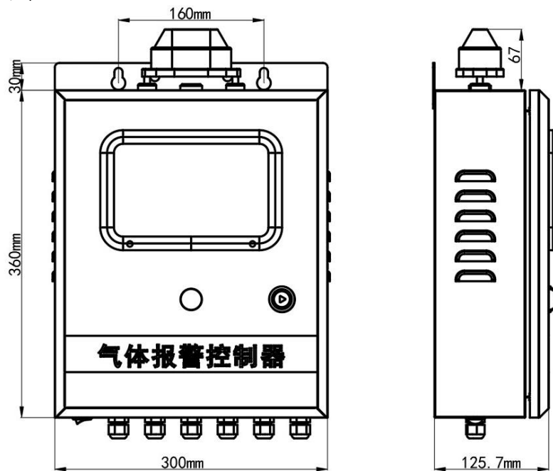
控制器尺寸 (单位 mm)
