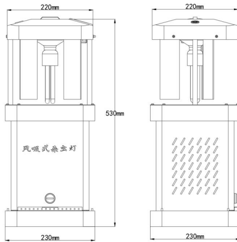
设备尺寸图 (单位: mm)
