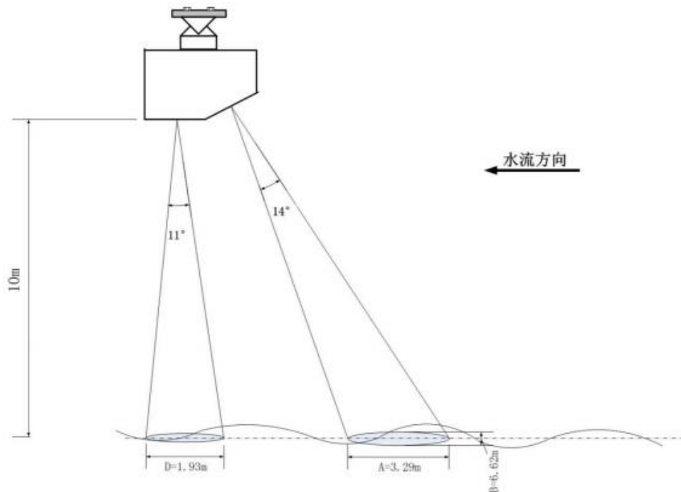
安装 10 米水位计和流速计天线照射区域
